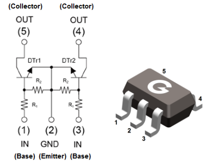
SOT-353
