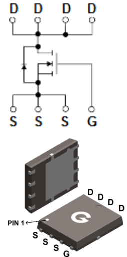
PDFN5x6-8L
