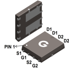
PDFN5x6-8LC
