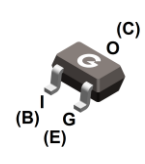
TDTB114EUA SOT-323
