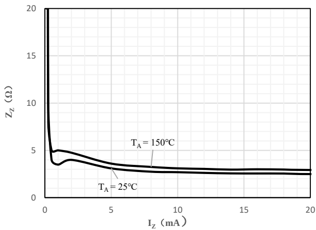
Fig 3 Zener Impedance vs. Zener Current
