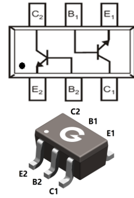
SOT-363
