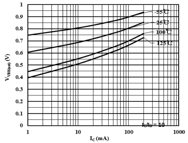
Fig 2 V_{BE(sat)} vs. I_C
