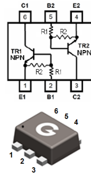
SOT-563
