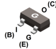
SOT-23-3L
