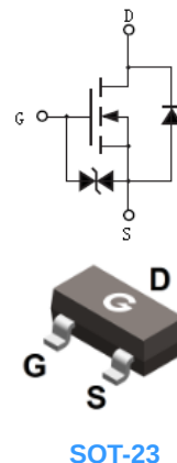
SOT-23
