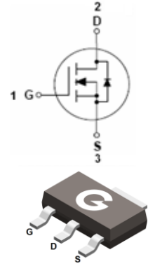
SOT-223
