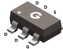
SOT-23-6L
