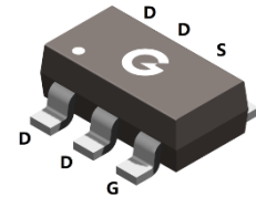
SOT-23-6L
