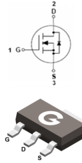
SOT-223
