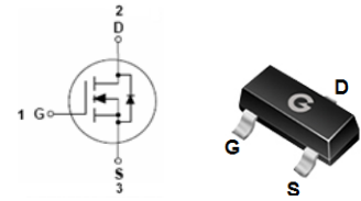
SOT-23
