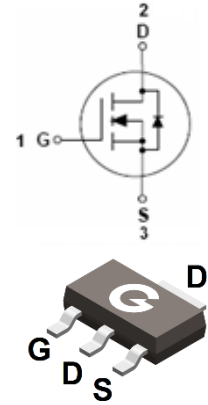
SOT-223
