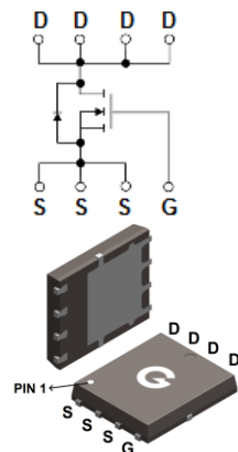
PDFN5×6-8L
