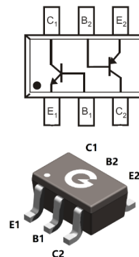
SOT-363
