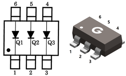
SOT-23-6L
