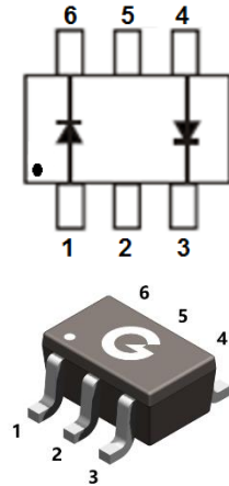
SOT-363
