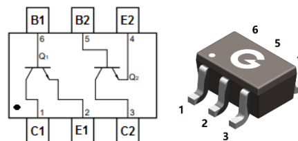
SOT-363
