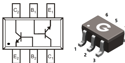
SOT-363
