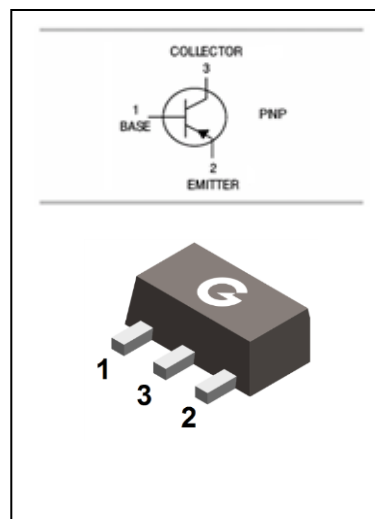
SOT-89
